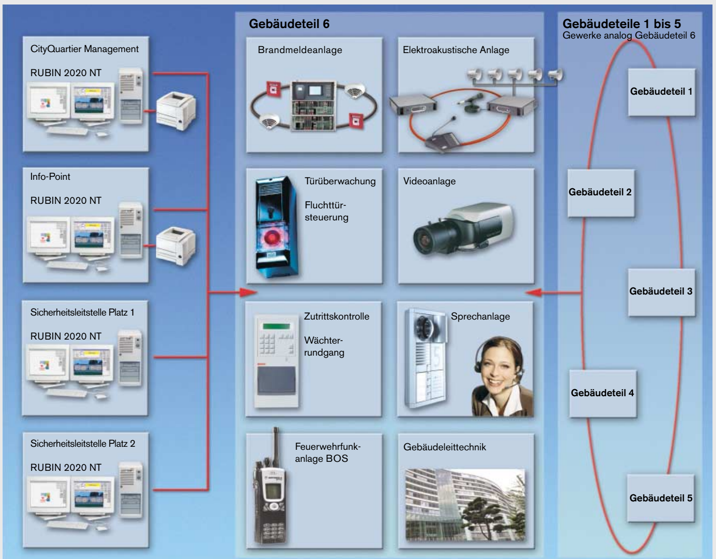
▲ Darstellung der miteinander vernetzten Gebäudeteile 1 bis 6 und ihrer installierten Systeme
